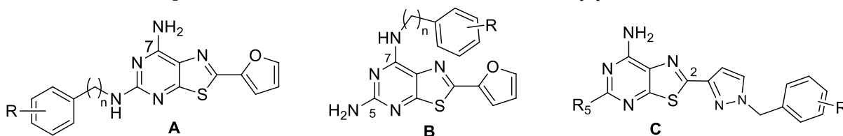
7-ammino-2-(furan-2-il)tiazolo[5,4-d]pirimidine
